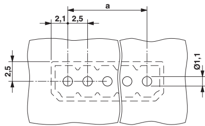
Bohrplan
