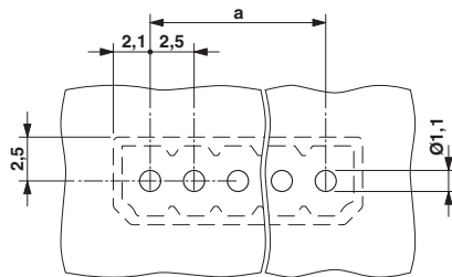
Bohrplan
