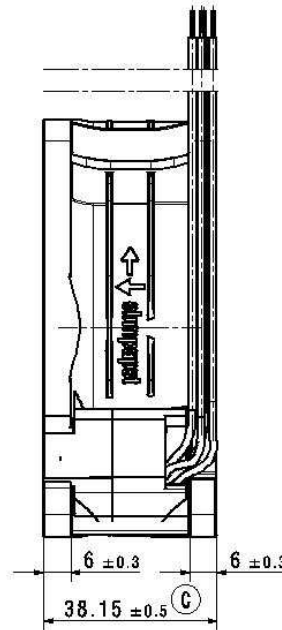
Seitenansicht links Maßstab: 1:1 side view left scale: 1:1
