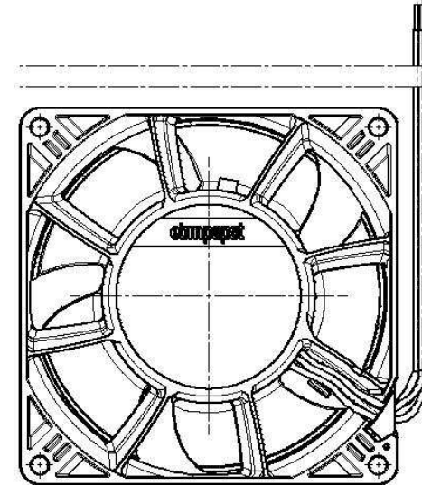
Rückansicht Maßstab: 1:1 back view scale: 1:1
