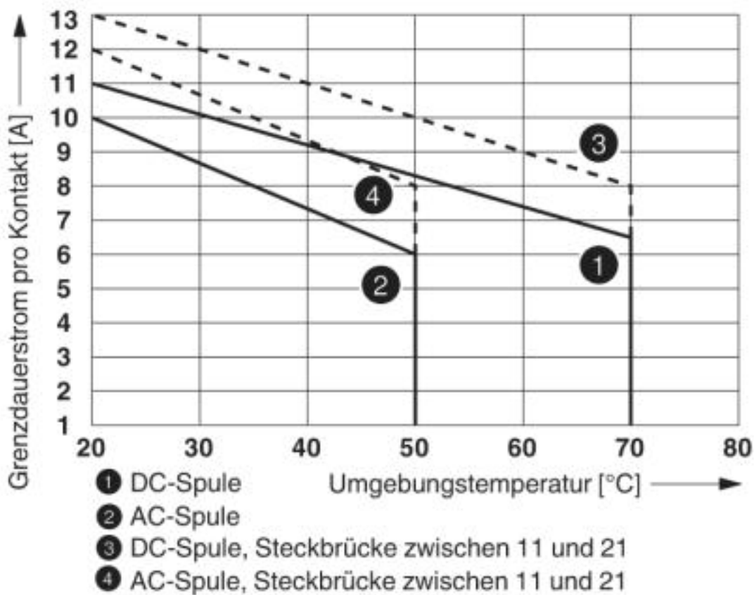
Kontaktderating
