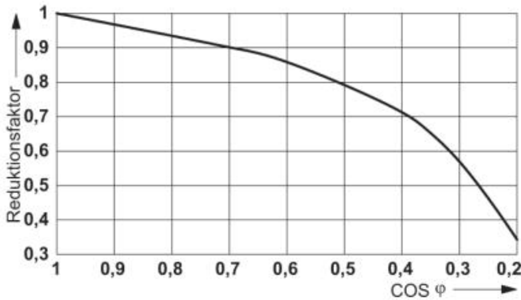
Lebensdauer-Reduktionsfaktor
