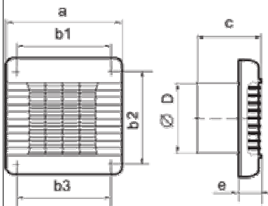
Abmessungen, mm
