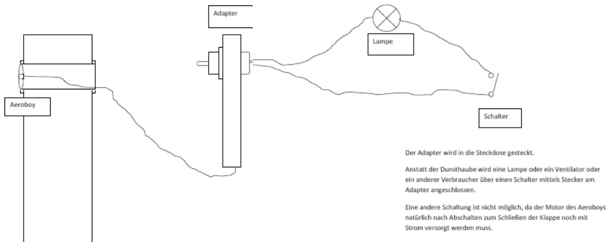
Skizze für Anschluss:
