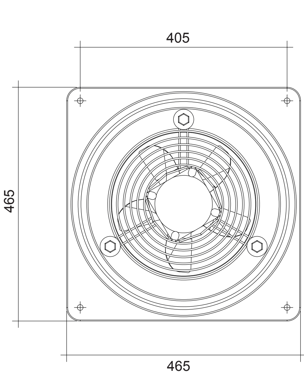
Außenwand-Ventilator BASIC 300 Material: Metall verzinkt
