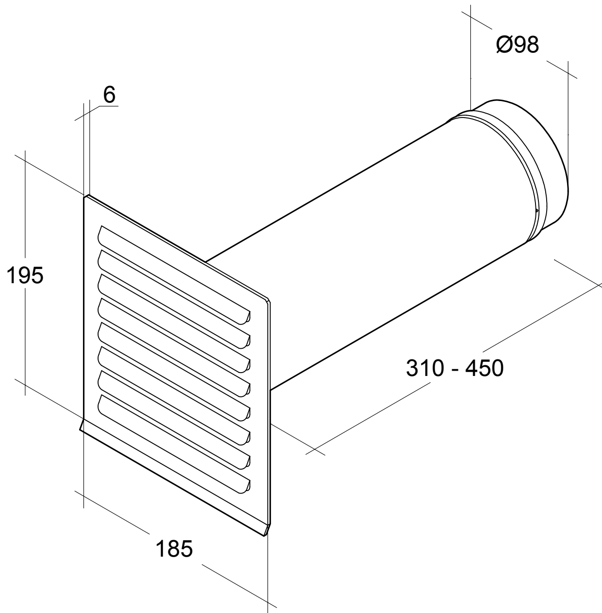
Teleskop-Rundrohrmauerkasten NW 100, m. RSK Material: verzinkt
