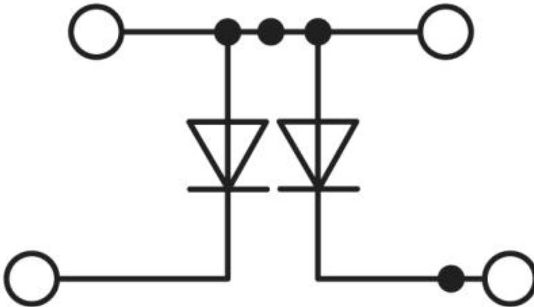
Schaltplan
