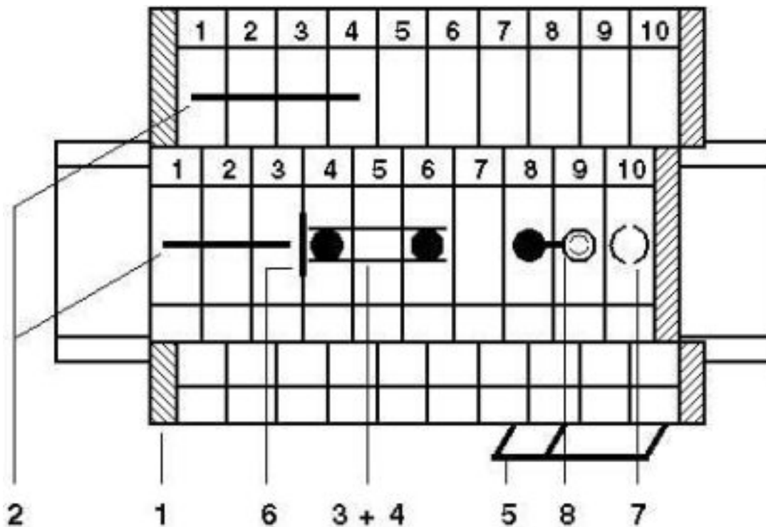
Schaltplan
