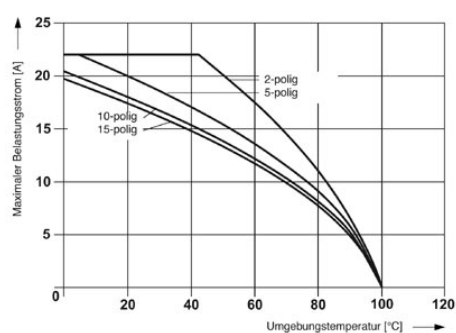
Deratingkurve für STTB 2,5/ 2P, STTB 2,5/ 2P-PV und für alle Steckervarianten SP... .
