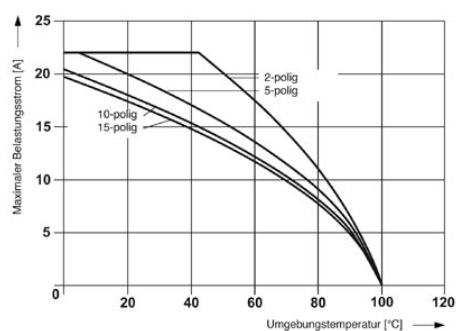
Deratingcurve für STTB 2,5/ 2P, STTB 2,5/ 2P-PV und für alle Steckervarianten SP... .
