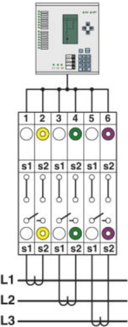
Einfacher Drei-Phasen-Stromwandlersatz
