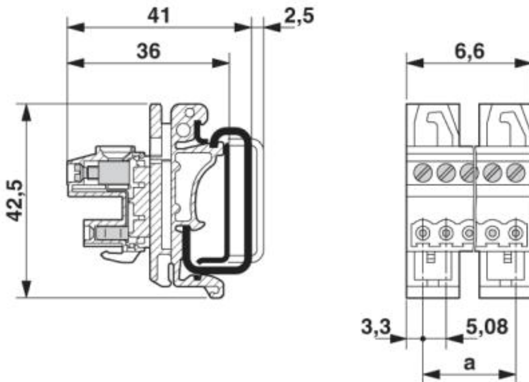
Maßzeichnung
