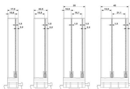
Detailmaßbild der Tragschienen- Busverbinder-Kontaktpads
