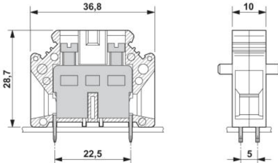
Maßzeichnung
