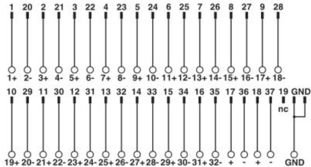
Anschlussbild VIP-2/.../D37SUB/M/SO
