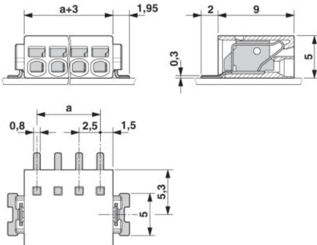
Maßzeichnung
