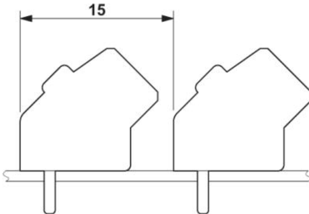
Maßzeichnung
