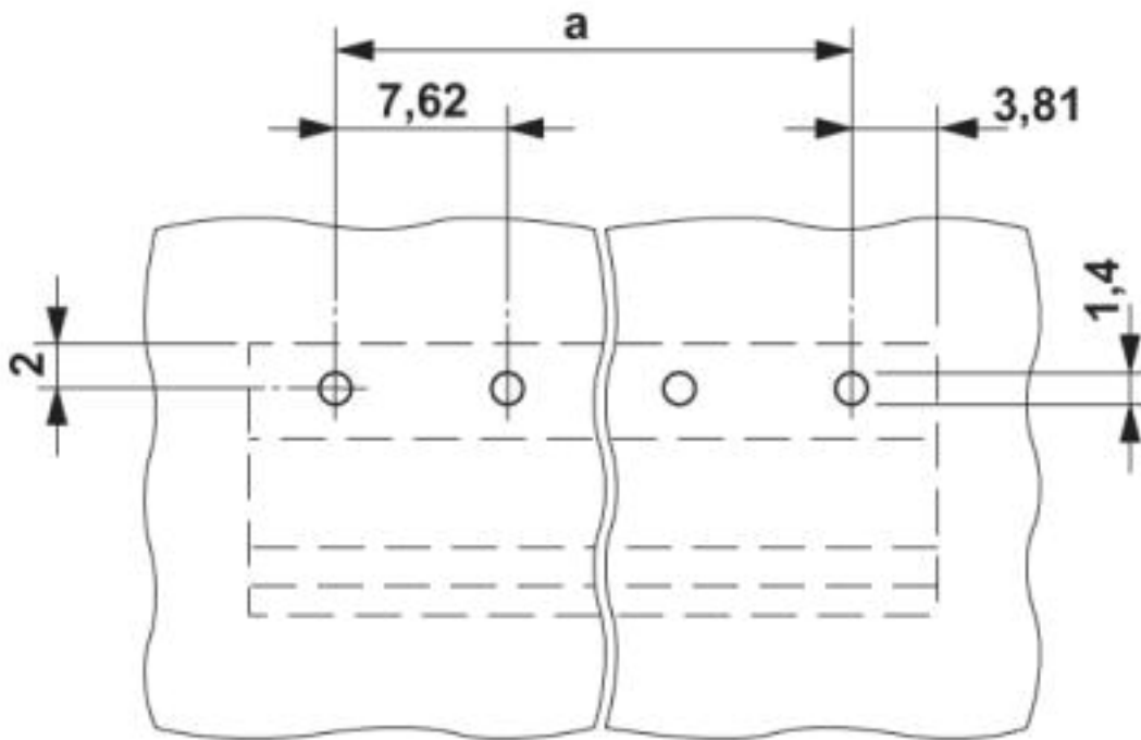
Bohrplan
