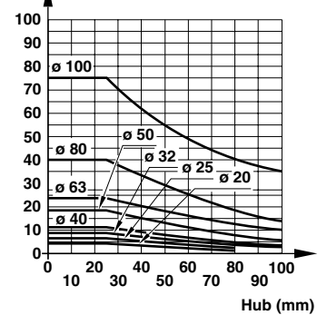
M - Drehmoment (Nm)
