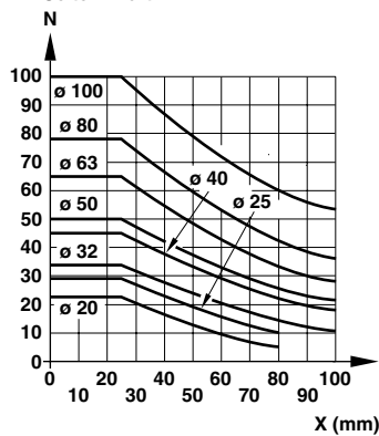
F - Seiten-Kraft
