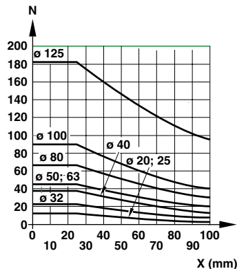
F - Seiten-Kraft
