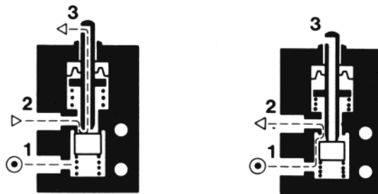
M/1553, Sperr-Nullstellung
