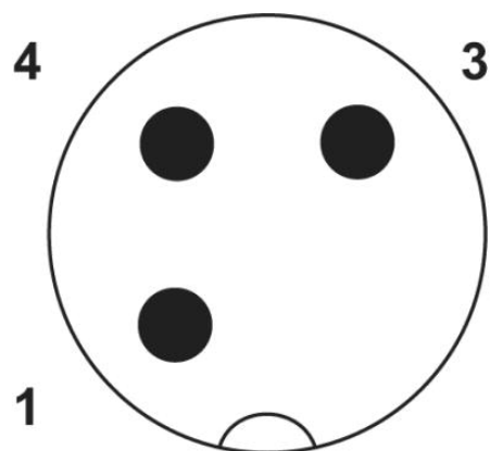
Polbild M12-Stecker, 3-polig, A-kodiert, Ansicht Stiftseite
