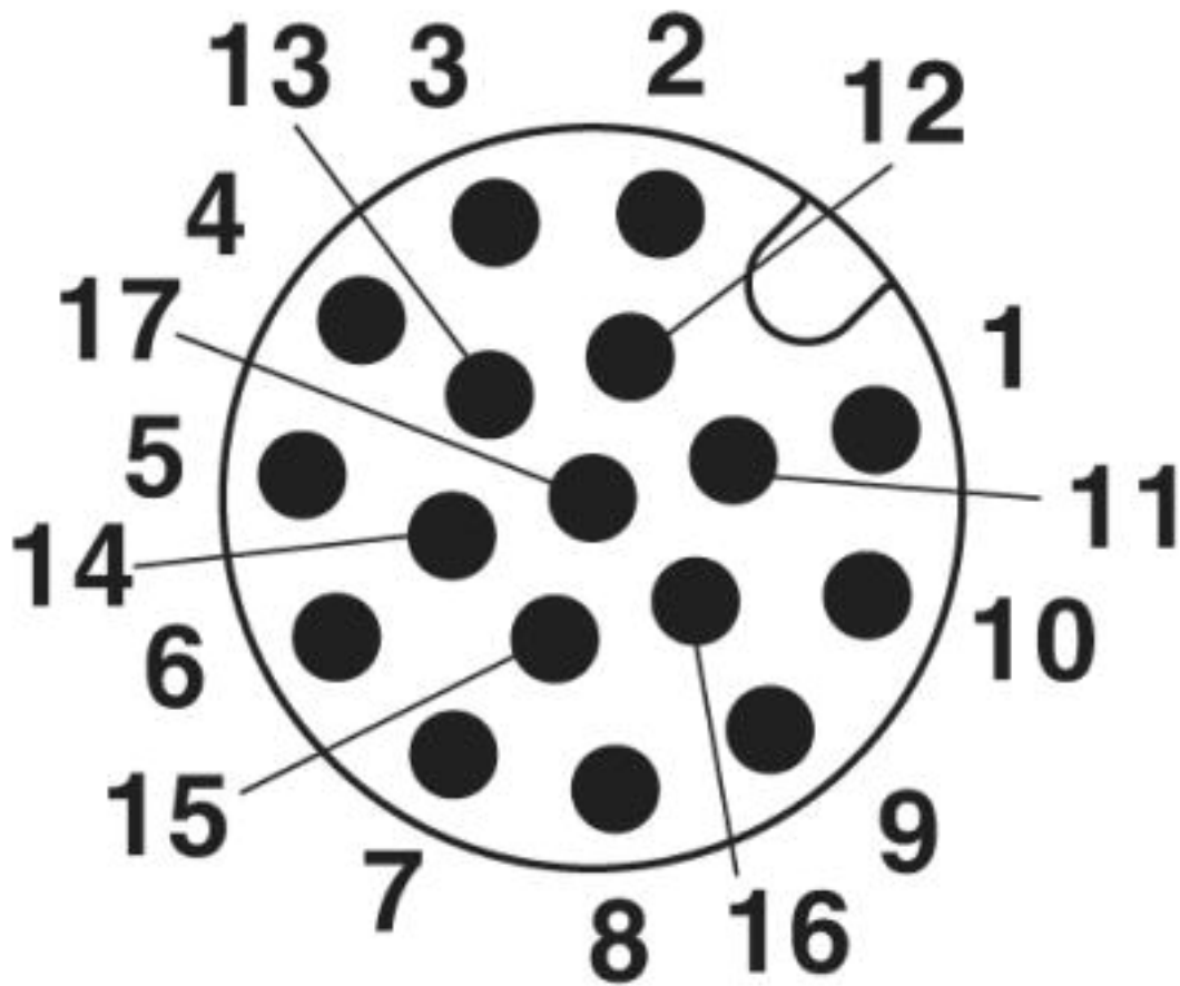
Polbild M12-Stecker, 17-polig, Ansicht Stiftseite
