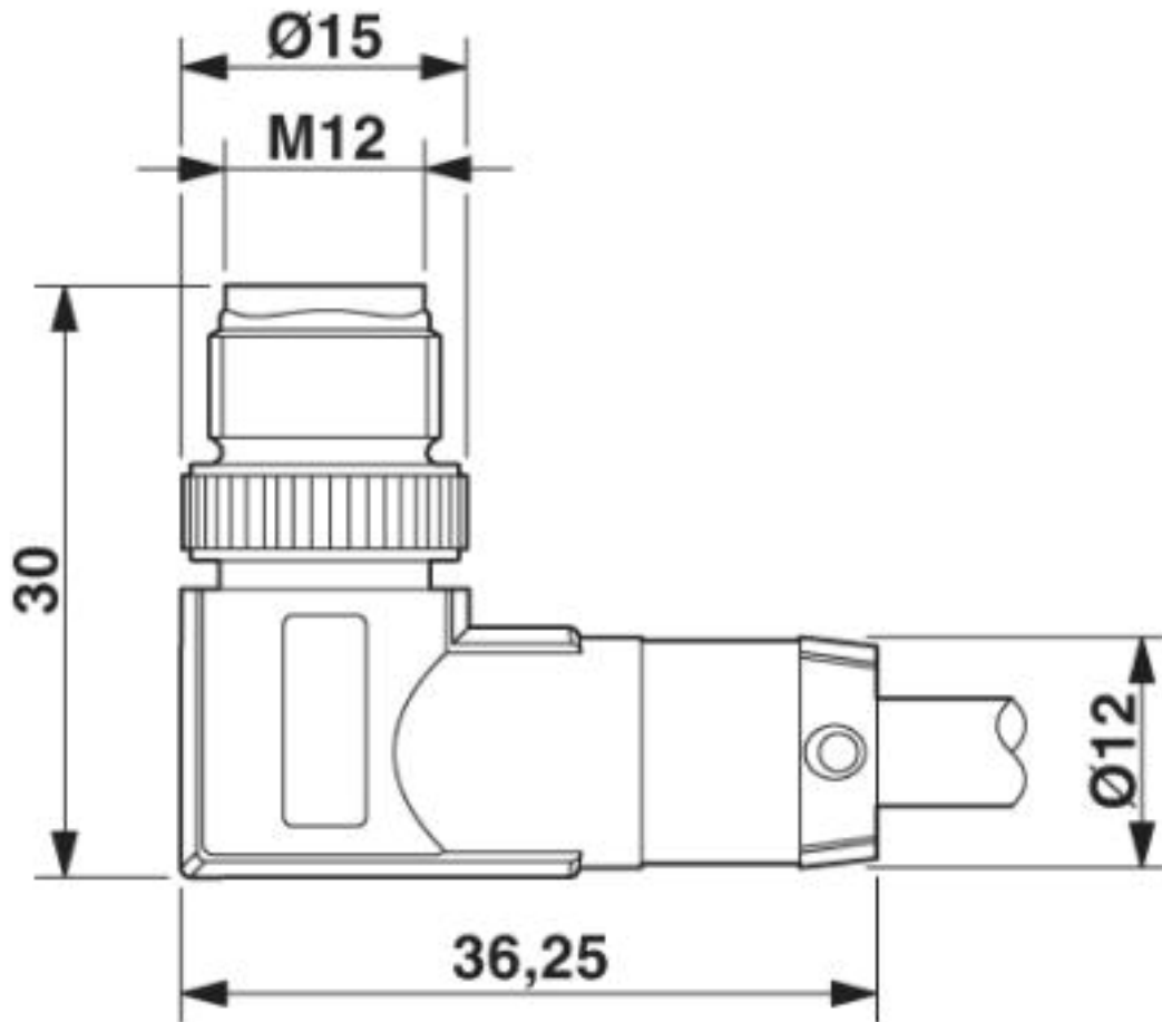
Stecker M12-SPEEDCON, gewinkelt
