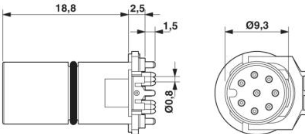
M12-Stift-Kontaktträger
