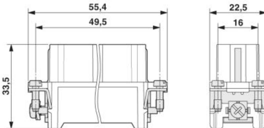
Buchseneinsatz
