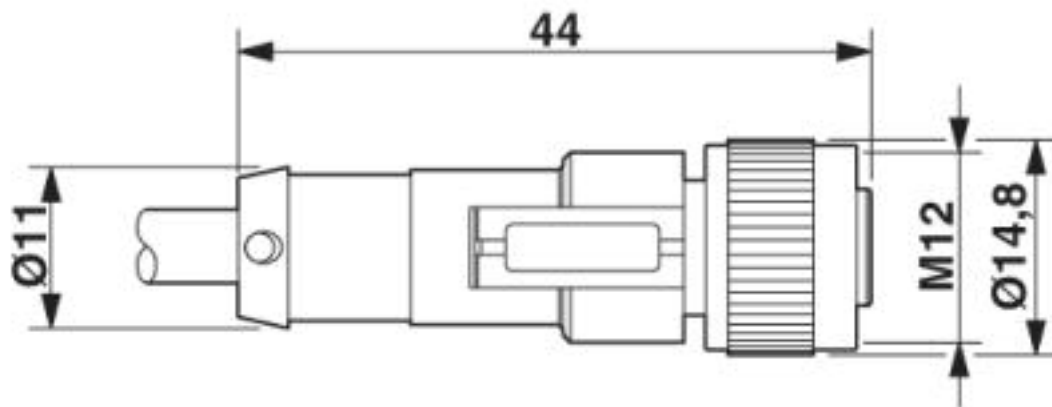
Buchse M12 x 1, gerade
