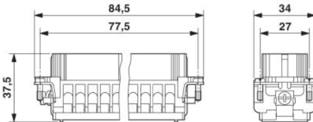
Buchseneinsatz
