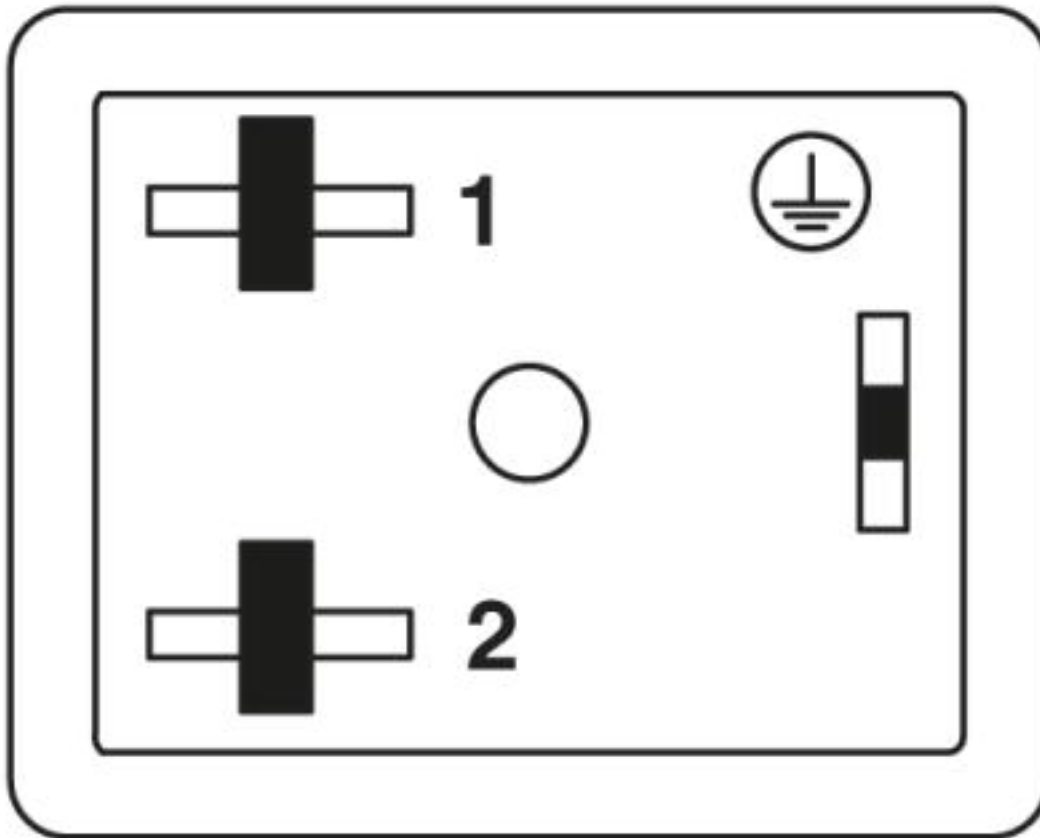
Polbild Ventilstecker, Bauform BI
