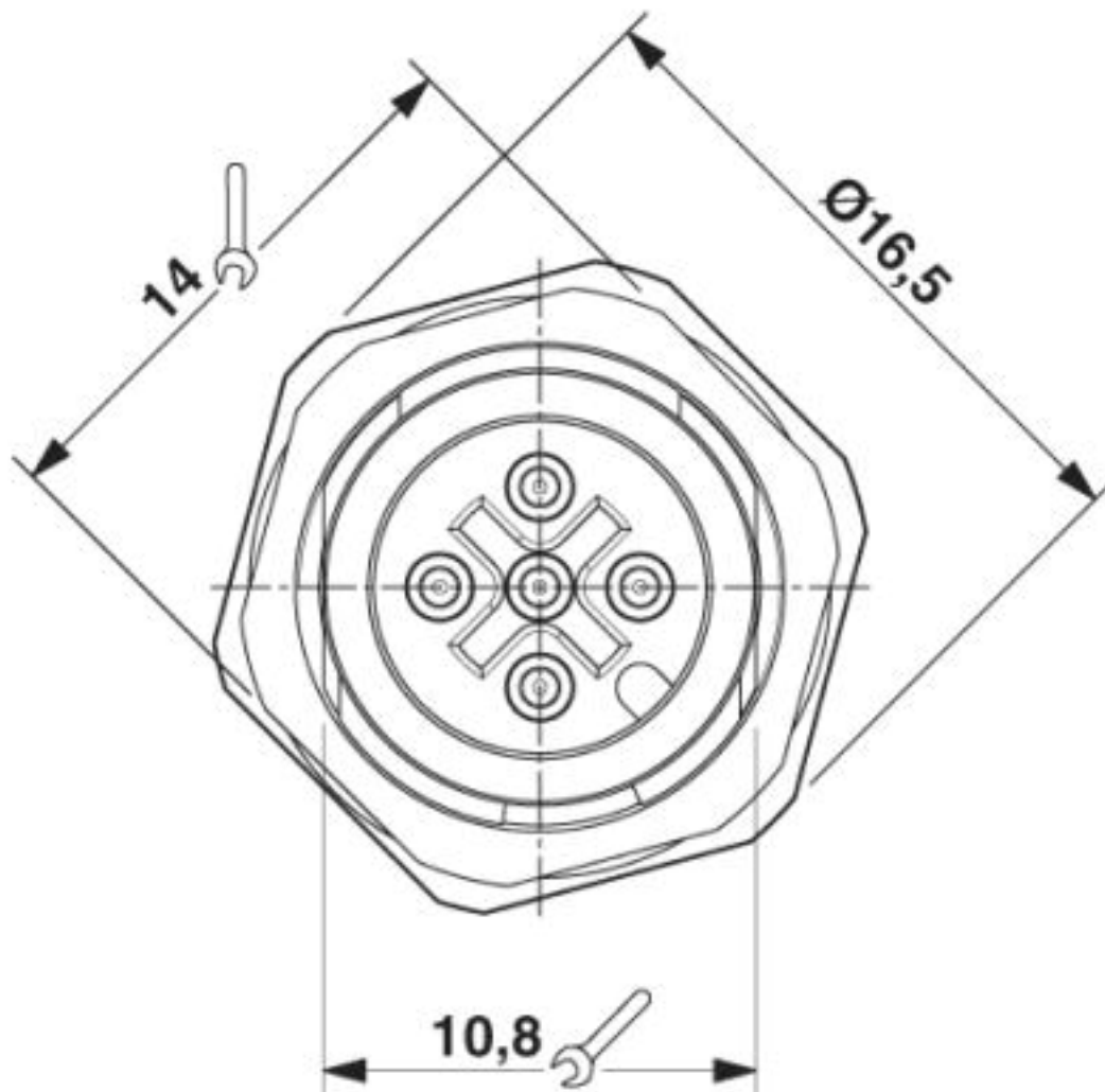
Frontansicht M12 Einbausteckverbinder
