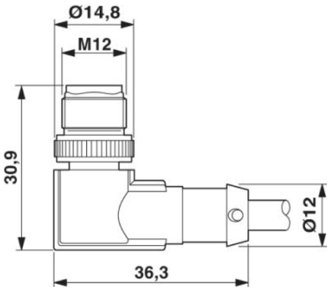
Stecker M12 x 1, gewinkelt, geschirmt
