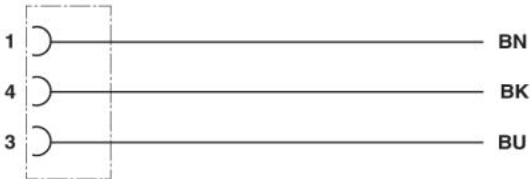
Kontaktbelegung der M8-Buchse
