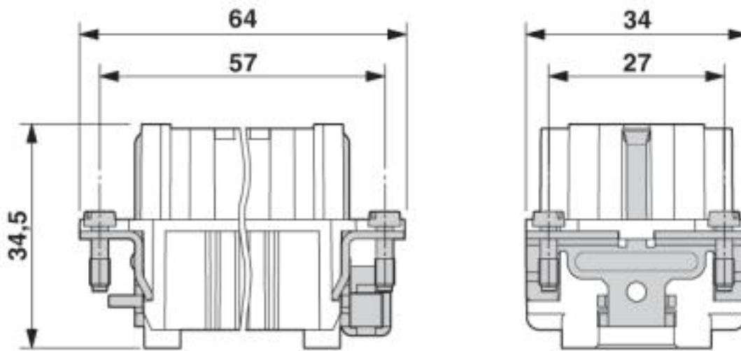
Buchseneinsatz
