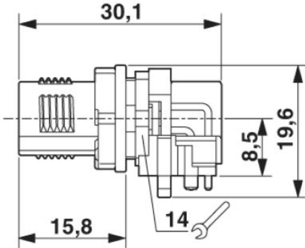
M12-Einbausteckverbinder, Stecker, Seitenansicht
