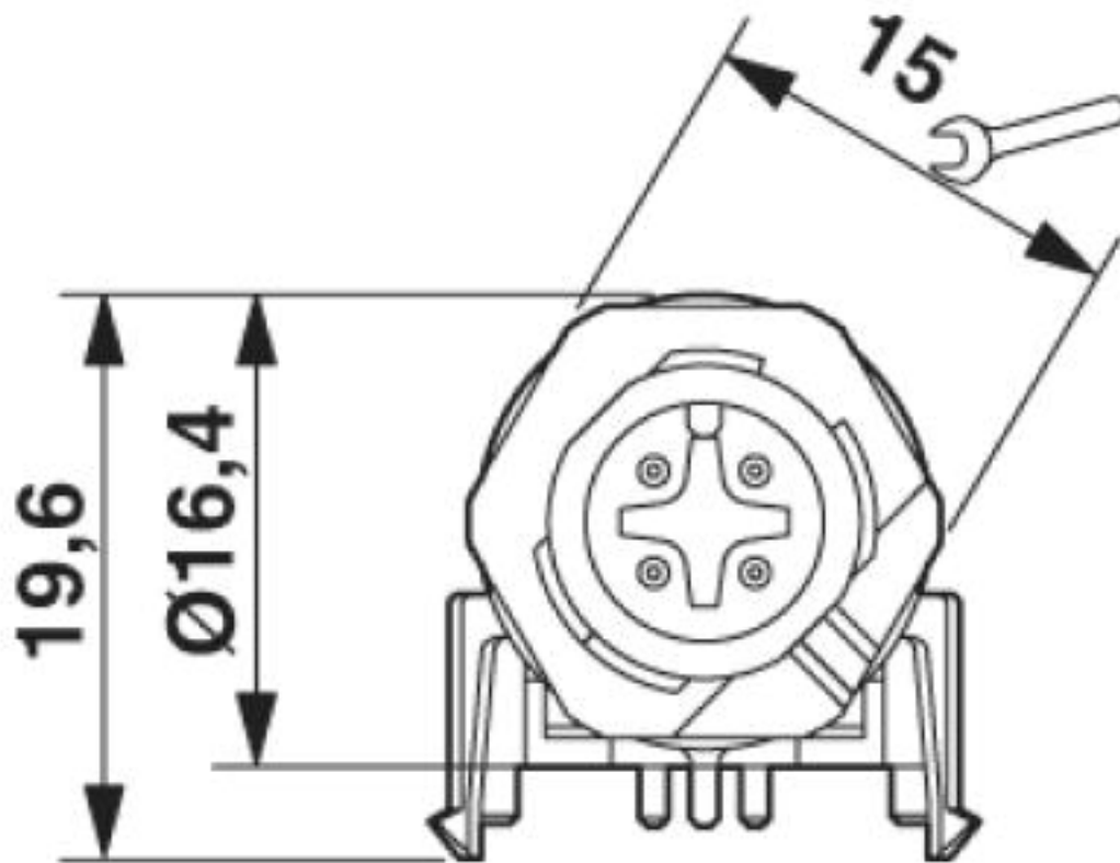
M12-Einbausteckverbinder, Stecker, Vorderansicht
