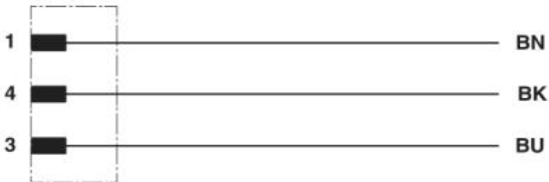
Kontaktbelegung des M12-Steckers
