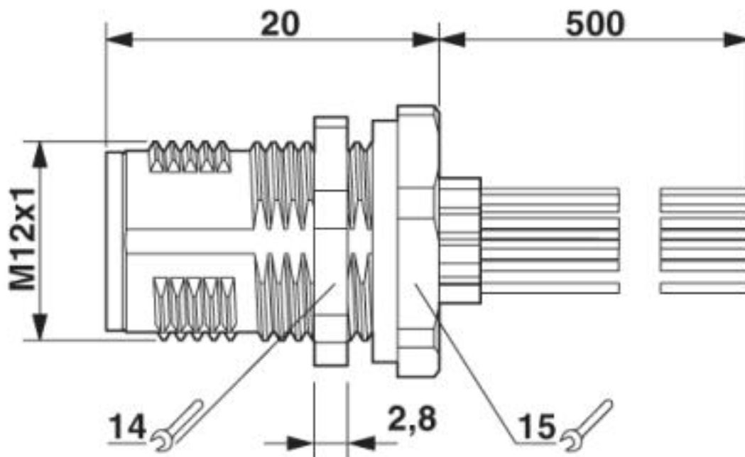
M12-Einbausteckverbinder
