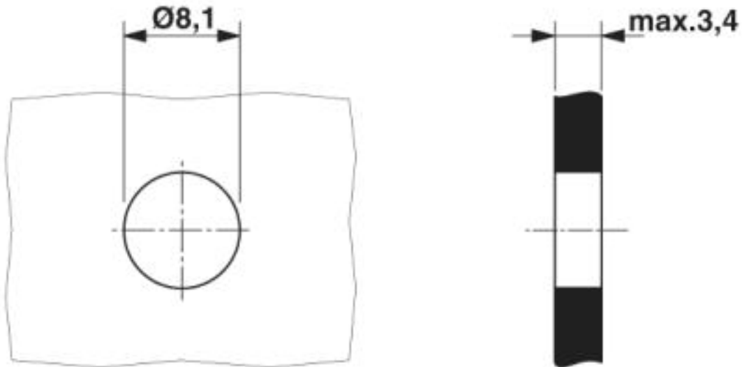
Gehäuseausschnitt für M8-Einbausteckverbinder, Stecker, einteilig
