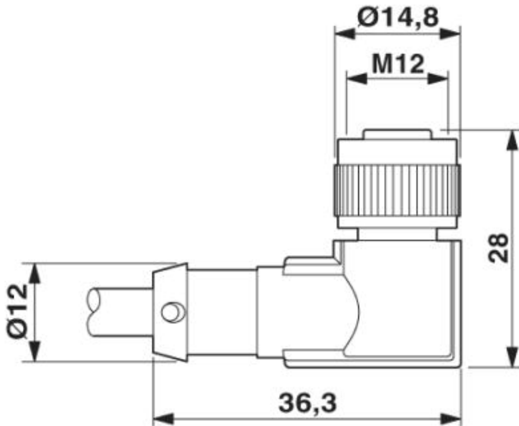
Buchse M12 x 1, gewinkelt, mit LED
