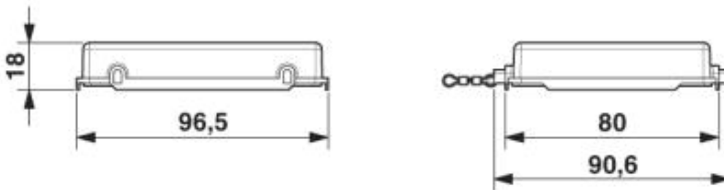
Schutzdeckel, B32
