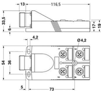
Maßzeichnung
