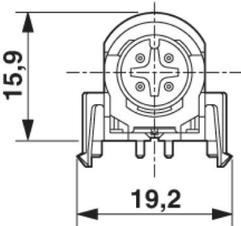
M12-Einbausteckverbinder, Stecker, Kontaktträger, Vorderansicht
