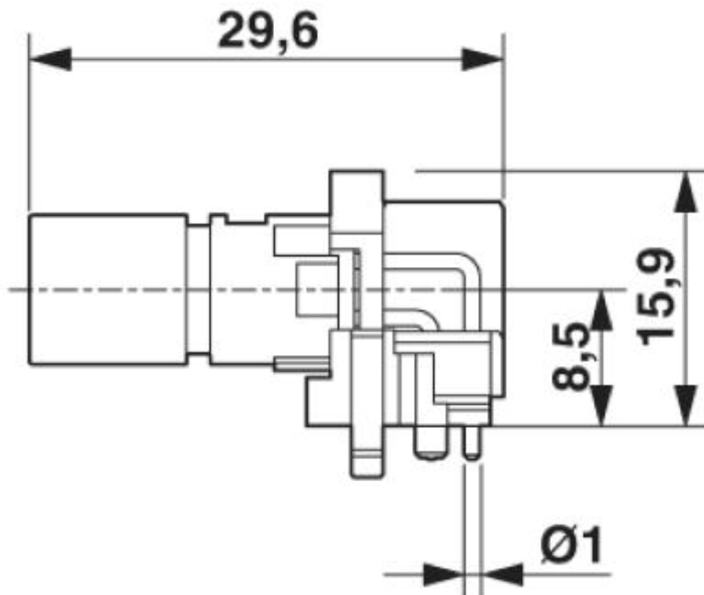
M12 Einbausteckverbinder, Stecker, Kontaktträger, Seitenansicht
