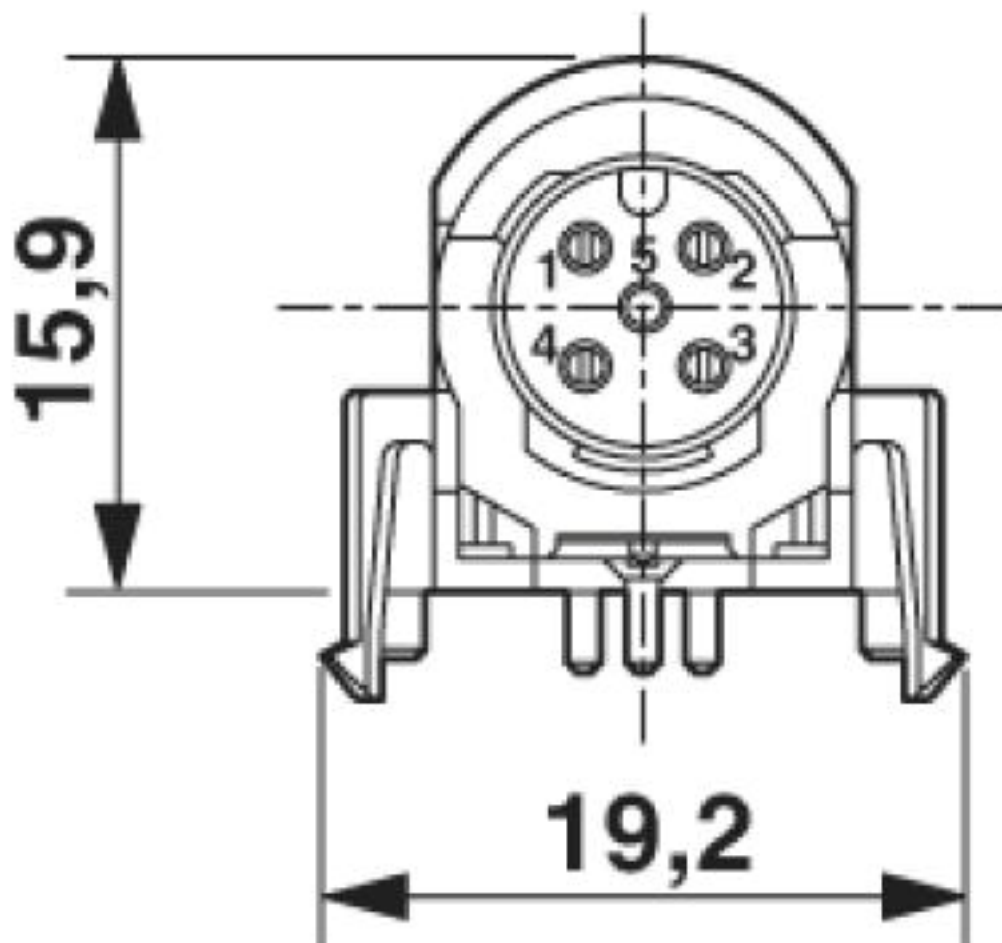
M12-Einbausteckverbinder, Buchse, Kontaktträger, Vorderansicht
