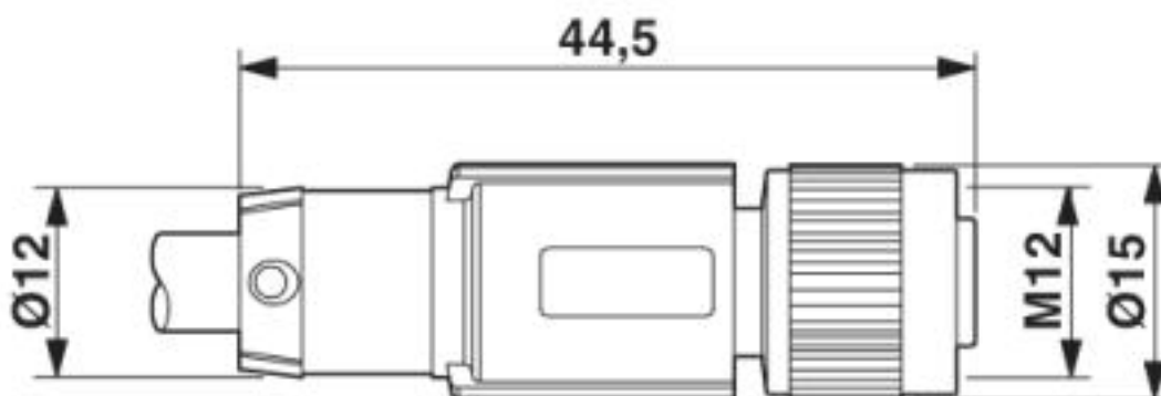
Buchse M12 x 1, gerade, geschirmt
