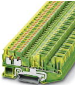
Schutzleiter-Reihenklemme, Anschlussart: Push-in- / Steckanschluss, Querschnitt: 0,14 mm 2 - 4 mm 2 , AWG: 26 - 12, Breite: 5,2 mm, Farbe: grün-gelb, Montageart: NS 35/7,5, NS 35/15
