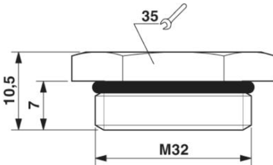
Blindstopfen M32
