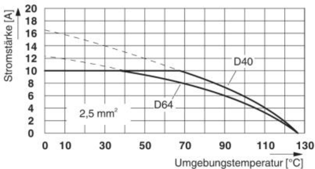
Deratingdiagramm für 2,5mm 2
