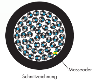
Schnittzeichnung
