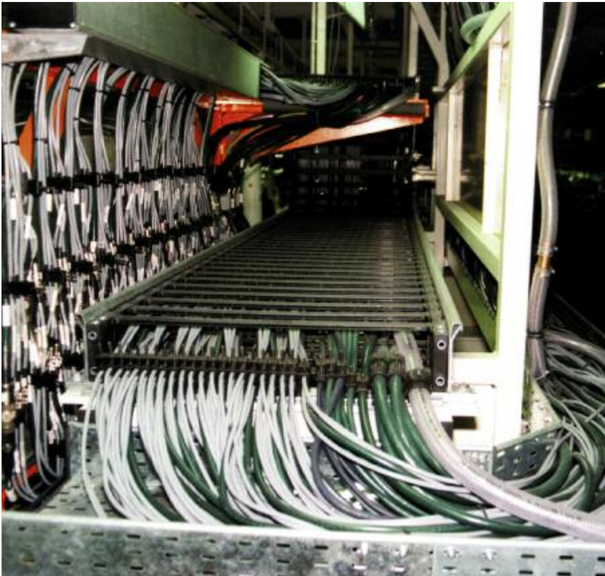
Chainflex® CF5 und CF6 Steuerleitungen (grün) sowie CF211 Messsystem-Leitungen (grau) in einer Schrauberstation im Automobilwerk. E-Kette® System E4/100 mit Chainfix Clip Zugentlastung.
