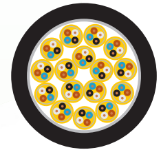
Schnittzeichnung
