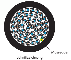
Schnittzeichnung
